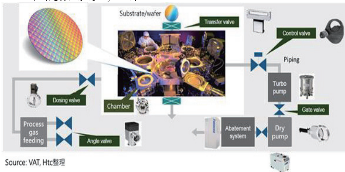
下圖是真空系統 layout 圖
